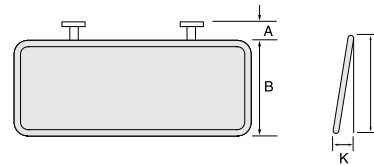
Ansicht T12/T13
